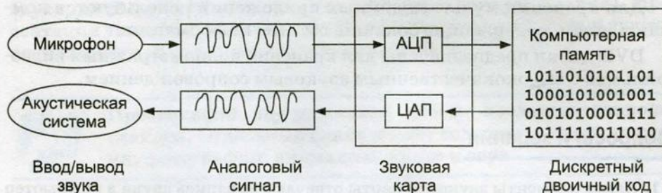
Рис. 5.3. Преобразование звука при вводе и выводе
