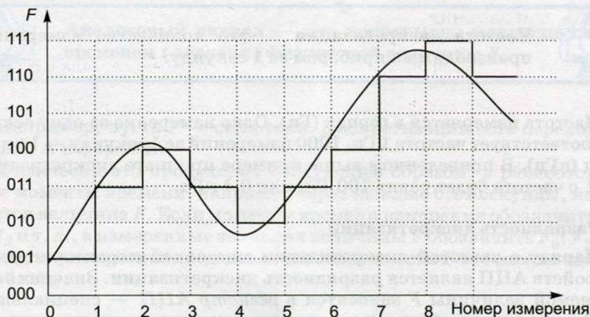
Рис. 5.8. Измерения переменной физической величины при использовании трехразрядного регистра
